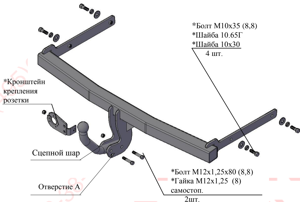
Рис.1 Тягово-сцепное устройство ТСУ 9711.
